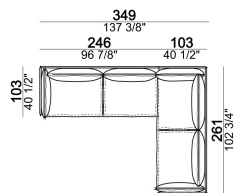
Composition "C" (élément gauche 246x103 cm + canapé d'angle gauche 261x103 cm)
